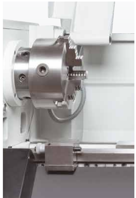
Der Mikrometer-Bettanschlag garantiert Wiederholgenauigkeit
