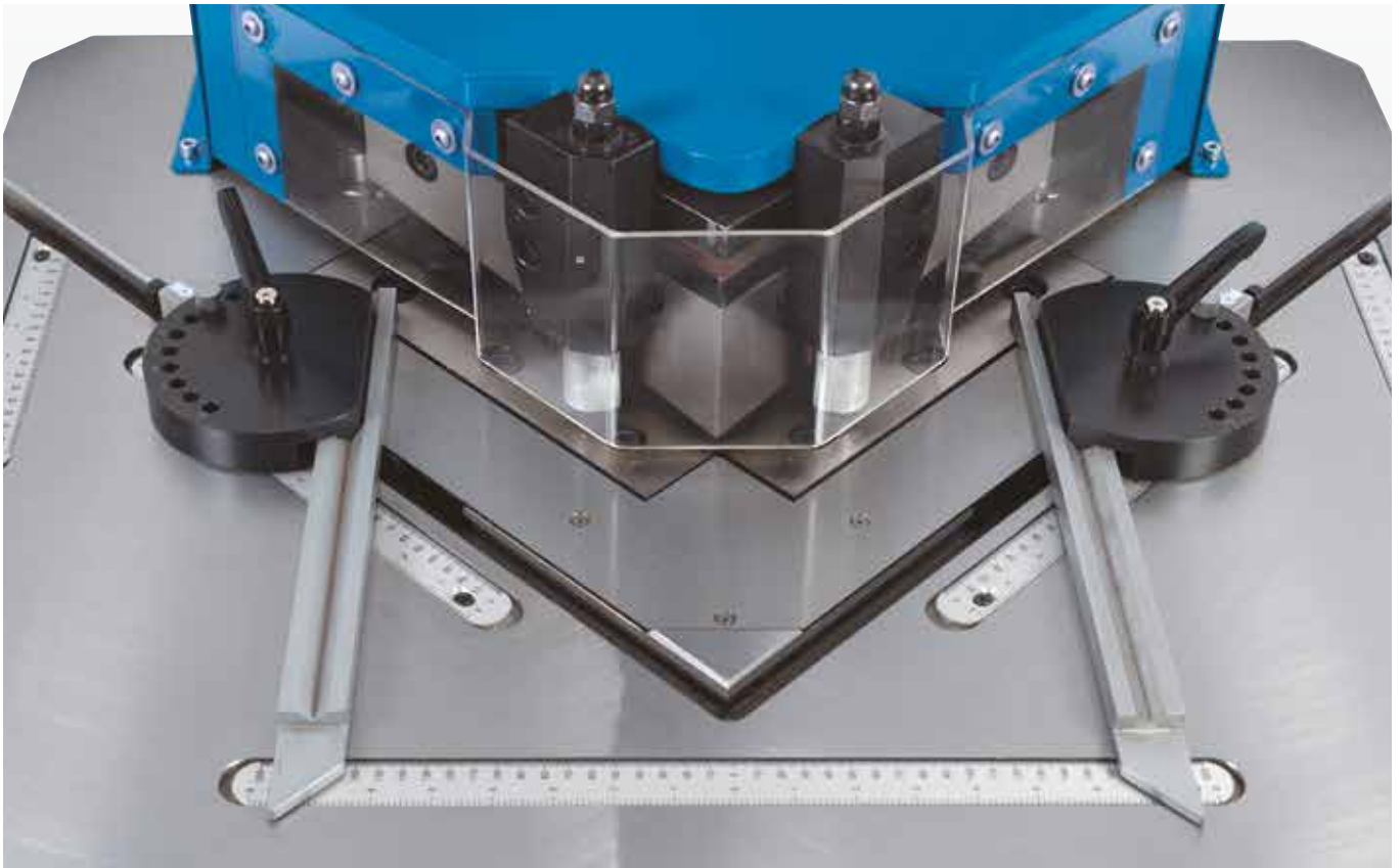
Maneta de fixare reglabila simplifica manipularea in siguranta a opririlor
