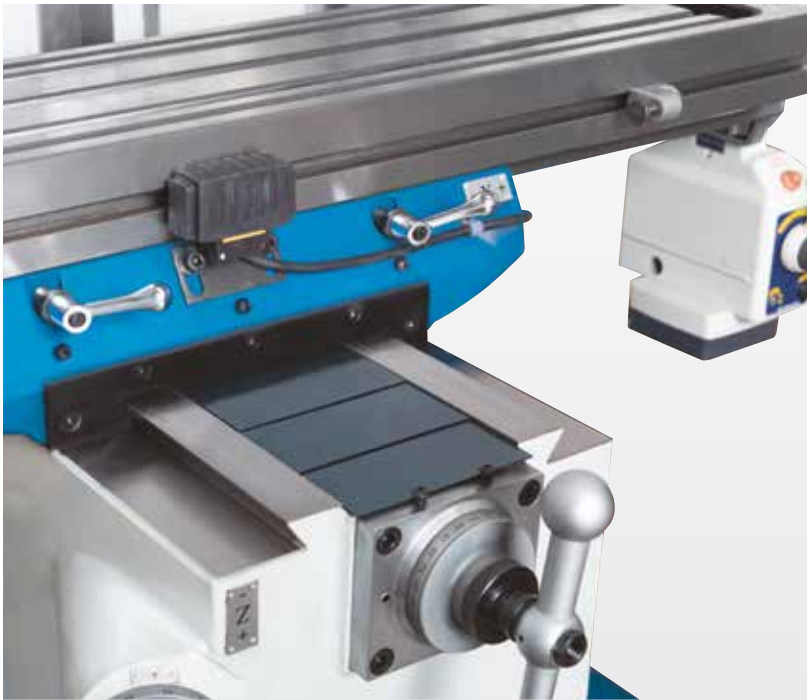
Ghidaje coadă de rândunică călite, reglabile în mod precis, în toate axele
